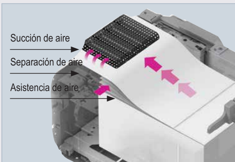
Las bandejas de papel LCT con alimentación de aire triple maximizan la confiabilidad y minimizan el tiempo de inactividad. Los sensores traumáticos mantienen un flujo de aire consistente.
