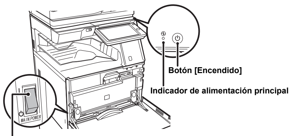
Interruptor de alimentación principal
